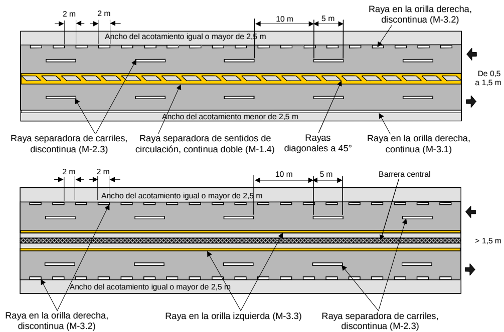
FIGURA 5.- Marcas en el pavimento en vialidades urbanas y carreteras de dos o más carriles por sentido de circulación
