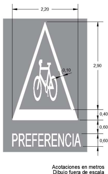
FIGURA 18.- Marca para vías ciclistas (M-15.2) con uso preferencial
