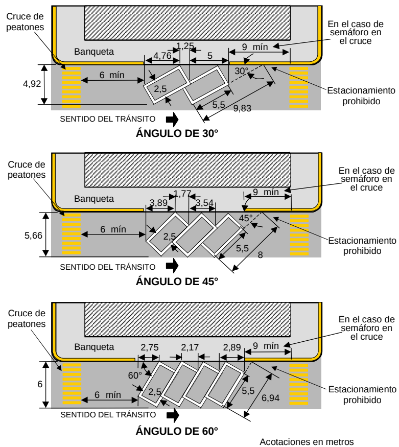
FIGURA 13.- Marcas para estacionamiento en batería
