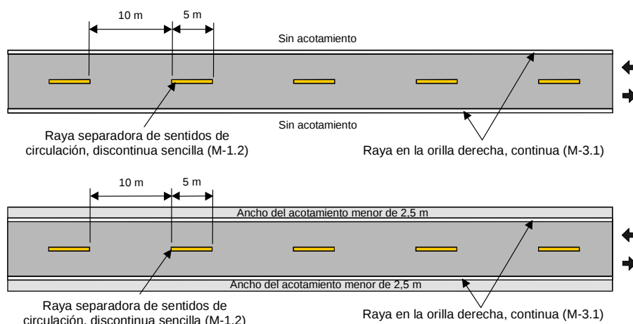
FIGURA 2.- Marcas en el pavimento en carreteras
