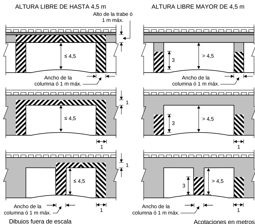
FIGURA 16.- Marcas en estructuras
