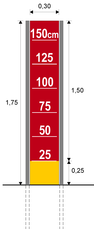
FIGURA 27.- Regla para vados y zonas inundables (OD-8)
