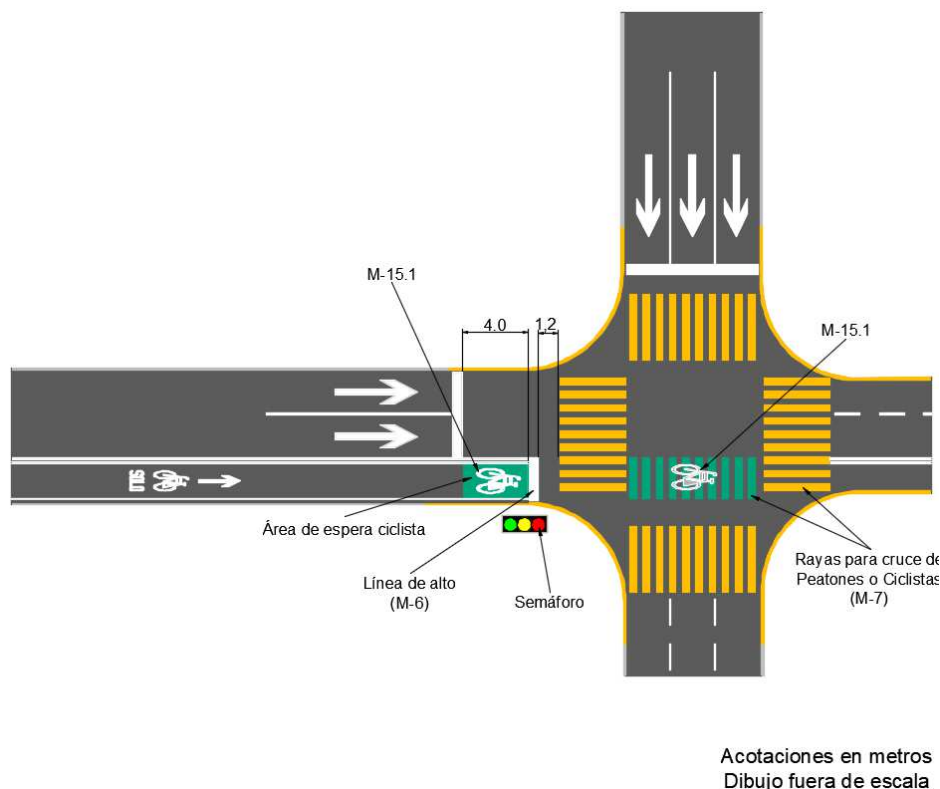
FIGURA 11.- Área de espera ciclista
