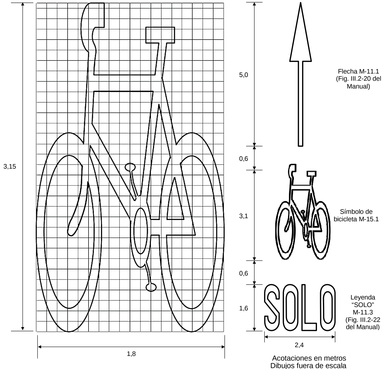
FIGURA 17.- Marcas para identificar vías ciclistas M-15.1
