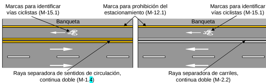
FIGURA 19.- Marcas para delimitar vías ciclistas
