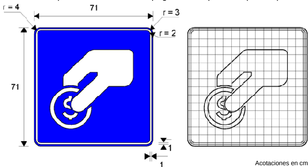
b) Módulo de pago (SIS-72)
