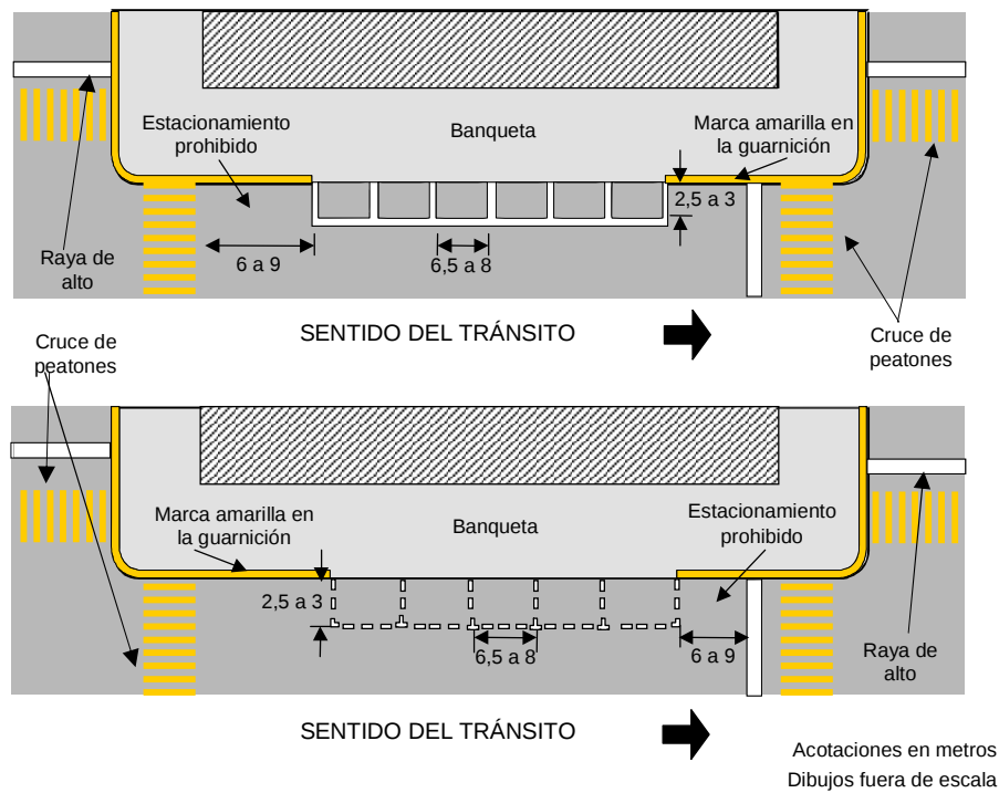
FIGURA 12.- Marcas para estacionamiento
