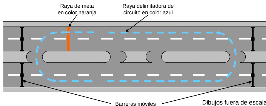
FIGURA 20.- Marcas temporales para circuito deportivo
