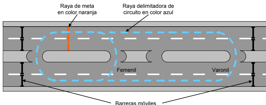
FIGURA 24.- Marcas para delimitar ciclovías
