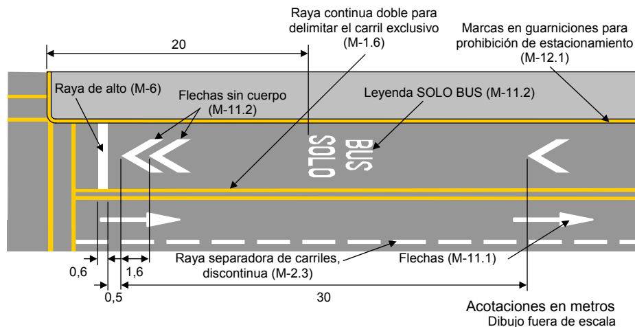
FIGURA 4.- Marcas para delimitar un carril en contrasentido
