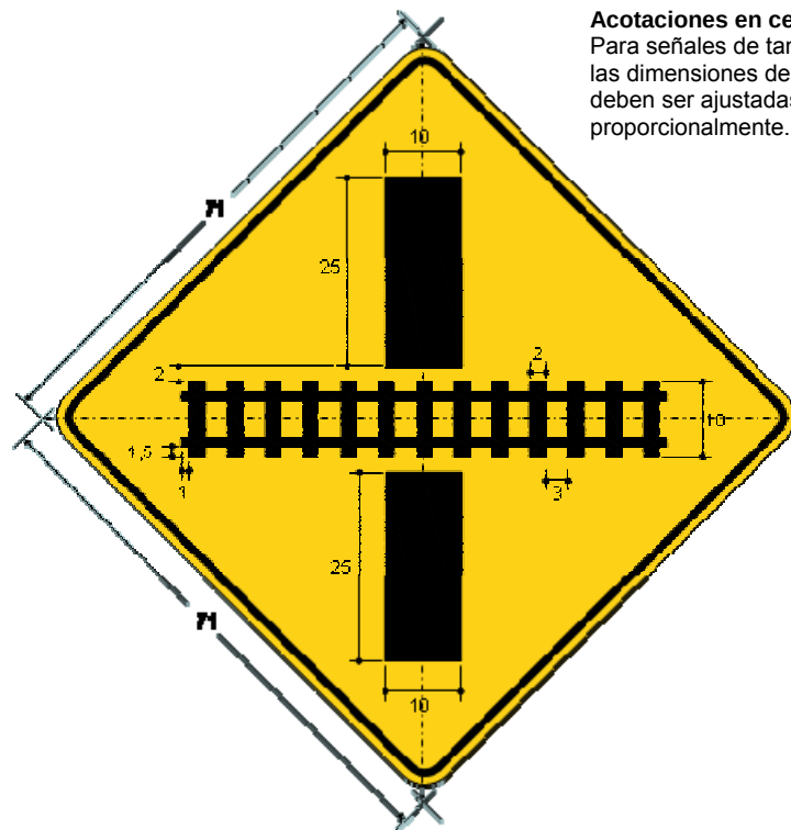
FIGURA B1.- SP-35 "Cruce con vía férrea" de 71 × 71 cm
