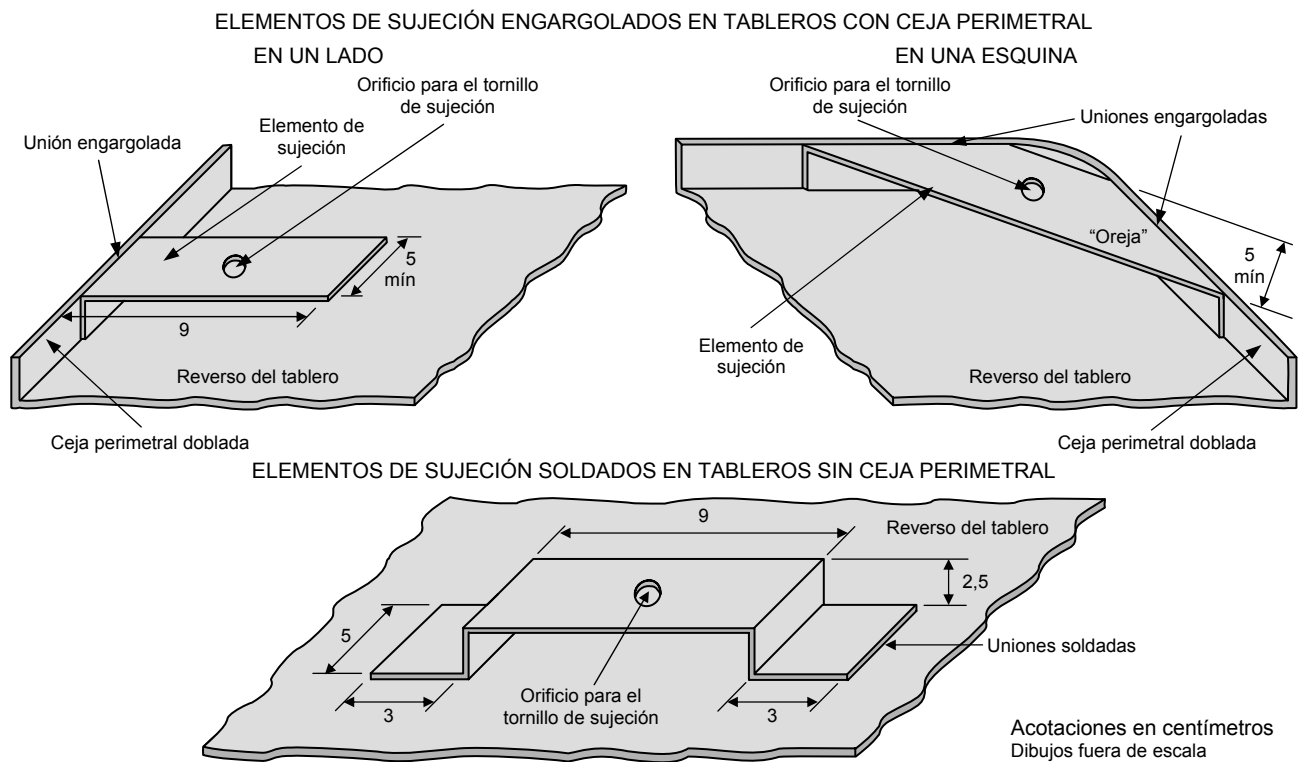
FIGURA 35.- Elementos de sujeción para señales bajas
