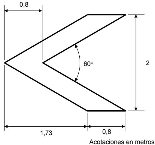
FIGURA 19.- Flechas sin cuerpo
