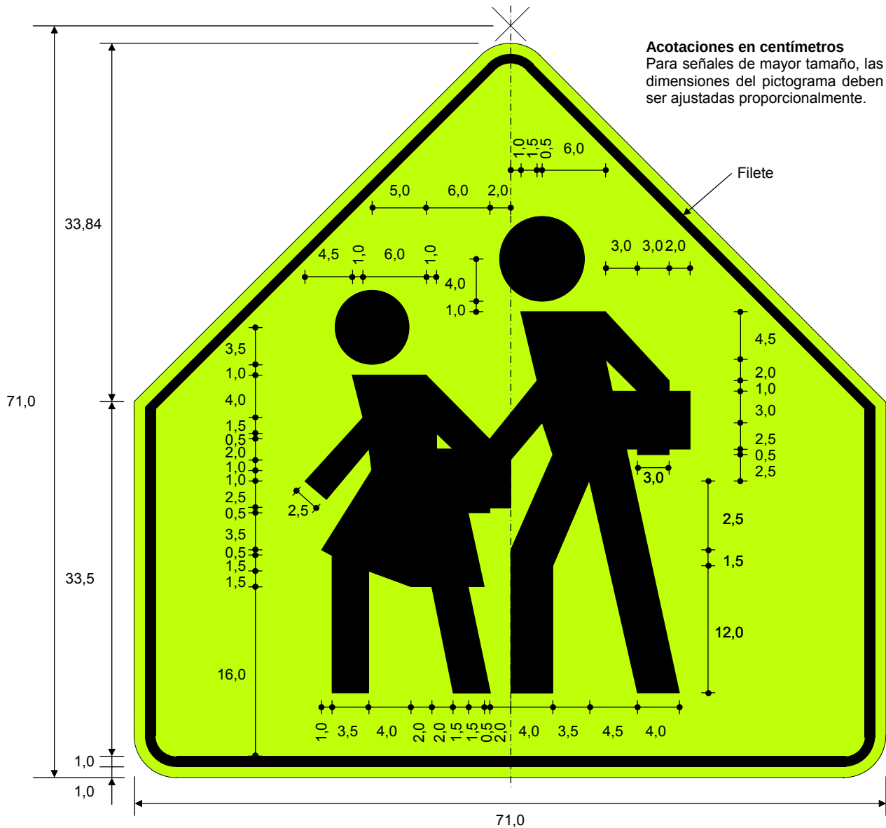
FIGURA 28.- Señal preventiva SP-33 "Escolares" de 71 × 71 cm
