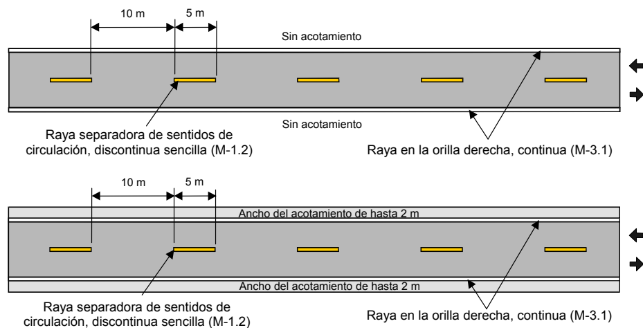
FIGURA 2.- Marcas en el pavimento en carreteras con ancho de arroyo vial de hasta 6,5 m
