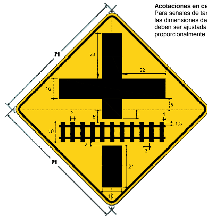
FIGURA B2.- SP-35A "Cruce con vía férrea y caminos" de 71 × 71 cm
