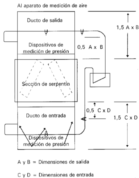
Figura A.8 - Medición de caída de presión estática del aire para una sección de serpentín sin ventiladores
