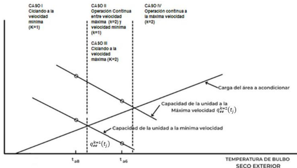
Figura 1a – Diagrama esquemático de varios modos de operación para la unidad INVERTER en modo frío
