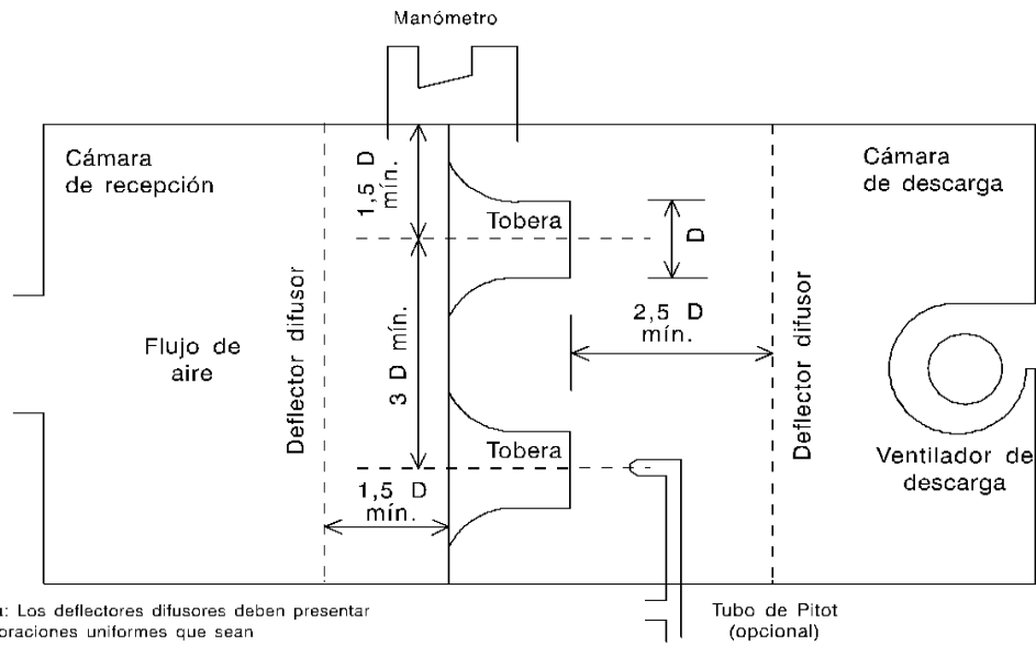
Figura A.5 - Aparato de medición de flujo de aire
