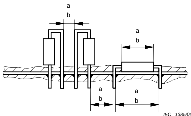
Figura 4b: placa con cables soldados que sobresalen
