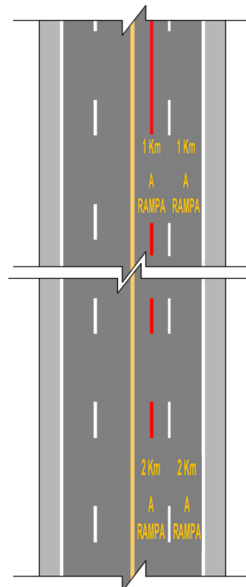
FIGURA 6.- Señalamiento horizontal de rampas de emergencia para frenado
