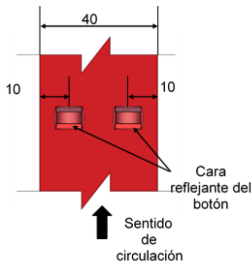
FIGURA 7.- Ubicación de los botones reflejantes
