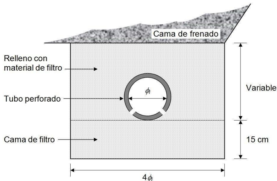
FIGURA 5.- Subdrén típico para la cama de frenado
