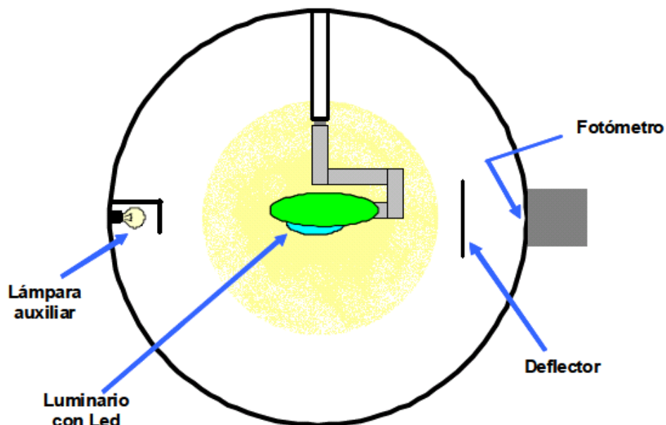
Figura F1. Configuración de la esfera integradora 4\pi
