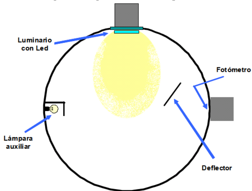
Figura F2. Configuración de la esfera integradora 2\pi
