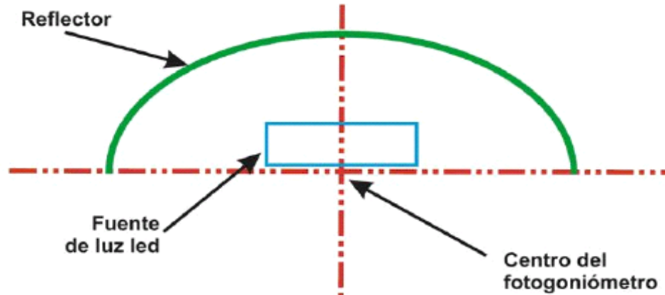
Figura D1. Montajes del luminario bajo prueba en el gonio-fotómetro
