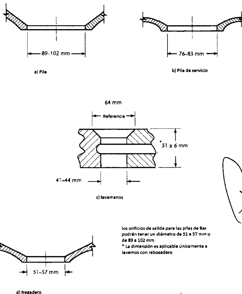
Figura 11.- Dimensiones de orificios de salida
