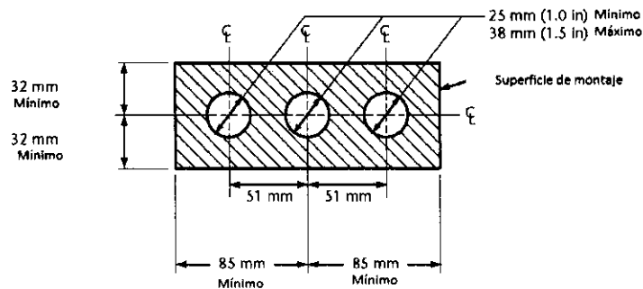
b) Griferías centrales normales de 100 mm
