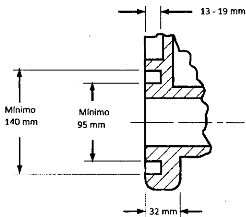
(a) taza de inodoro de colgar con orificio de salida trasero.
