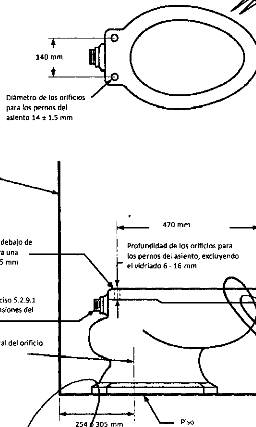
(b) Inodoro con orificio trasero y orificio de salida inferior
