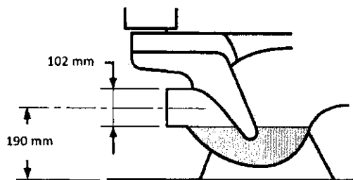
(c) Taza de inodoro para instalar en el piso con orificio de salida de espiga trasera.
