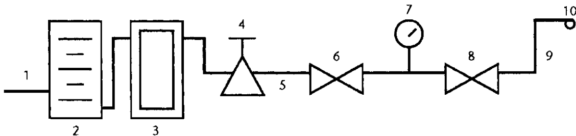
a) Sistema de suministro de agua tipificado
