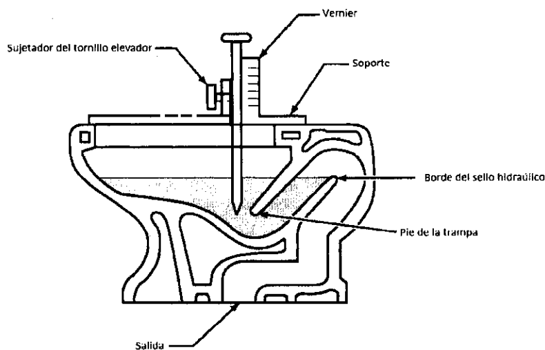
a) Aparato sugerido
