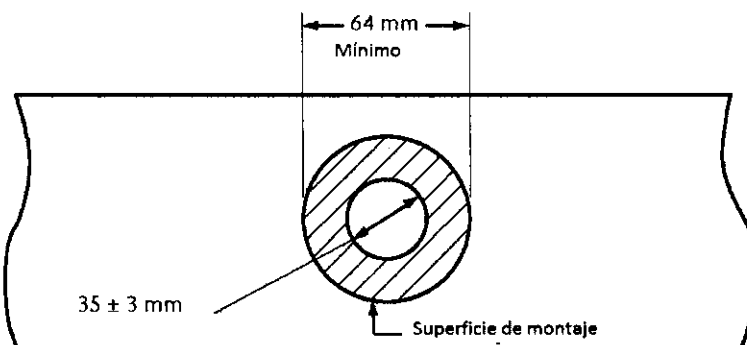
c) Grifería de montaje sencillo
