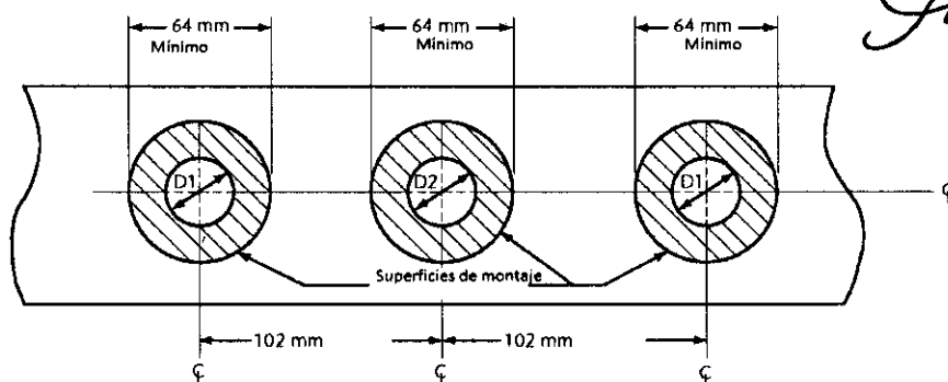
a) Griferías de combinación normales de 200 mm
