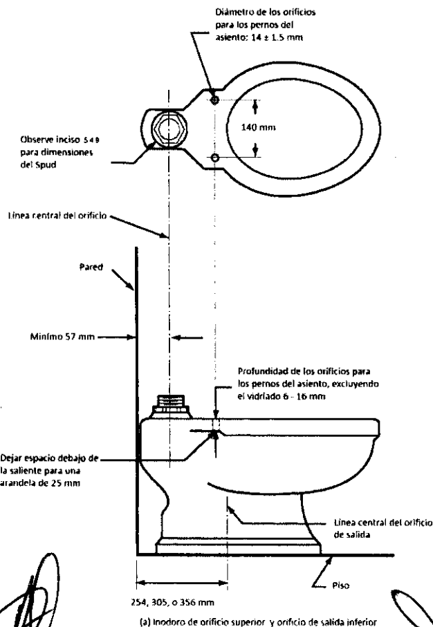
(a) Inodoro de orificio superior y orificio de salida inferior
