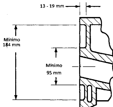
(d) Taza de inodoro para instalar en el piso con orificio de salida trasero
