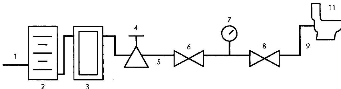
b) sistema de suministro de agua tipificado listo para las pruebas de inodoros
