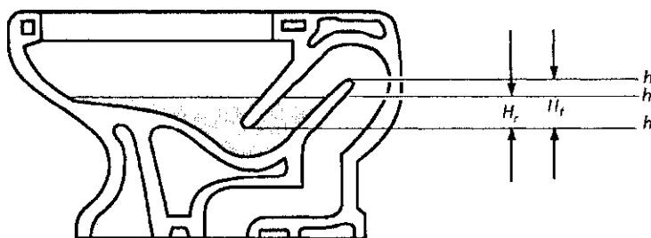
b) Mediciones requeridas
