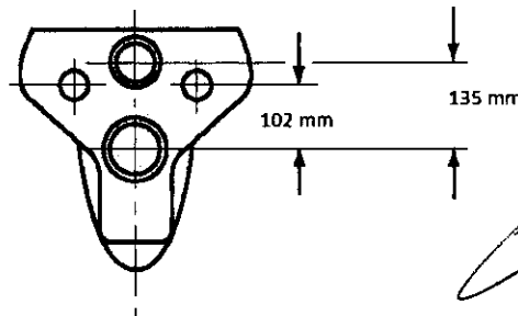
(b) inodoro de colgar con taza no sifónica y orificio de salida trasero.
