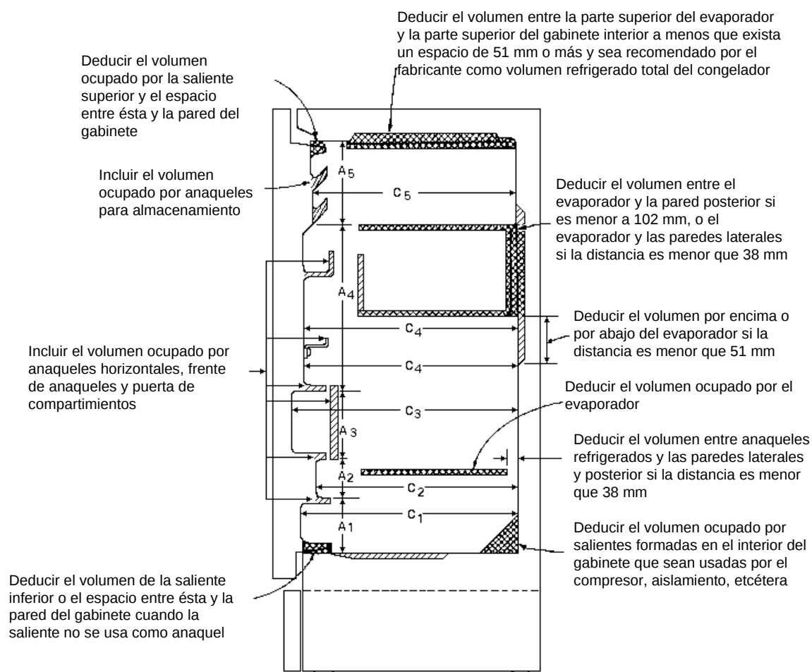
Figura 18. Congelador vertical
