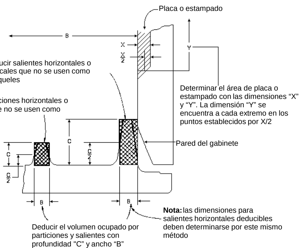
Figura 23. Saliente de la puerta y dimensiones lineales de la placa
