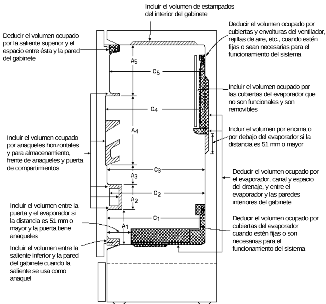
Figura 19. Congelador vertical
