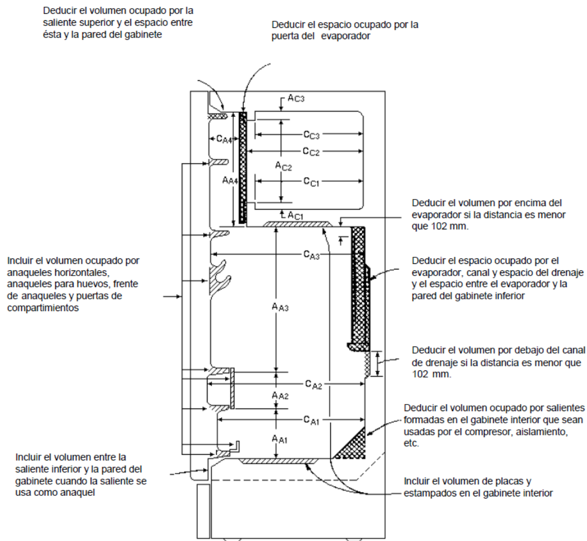
Figura 7. Refrigerador convencional
