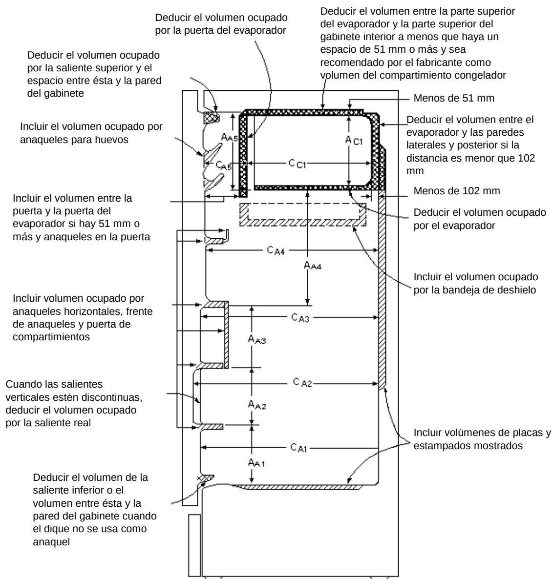
Figura 6. Refrigerador convencional
