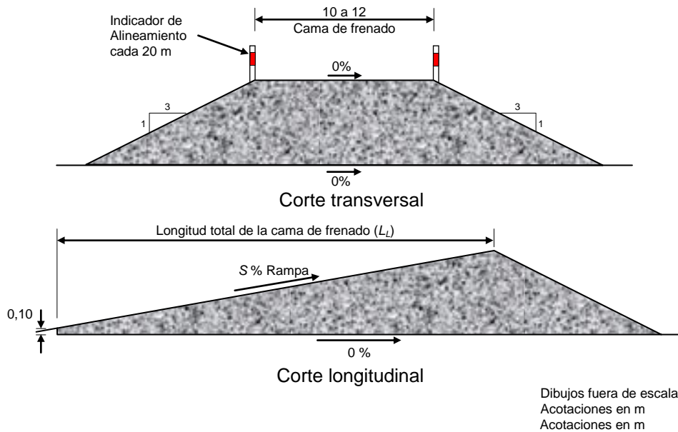
Figura 3.- Disposición en corte de las rampas de emergencia para frenado tipo RE-1
