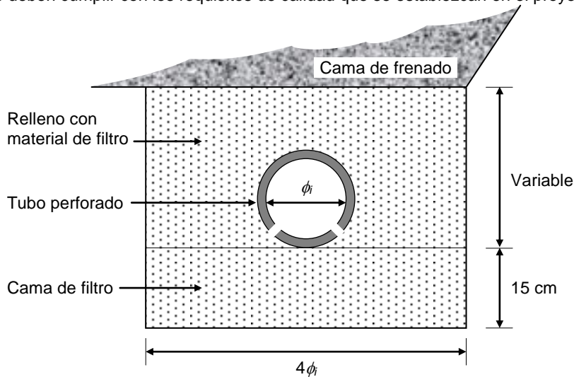
Figura 6.- Subdrén típico para la cama de frenado
